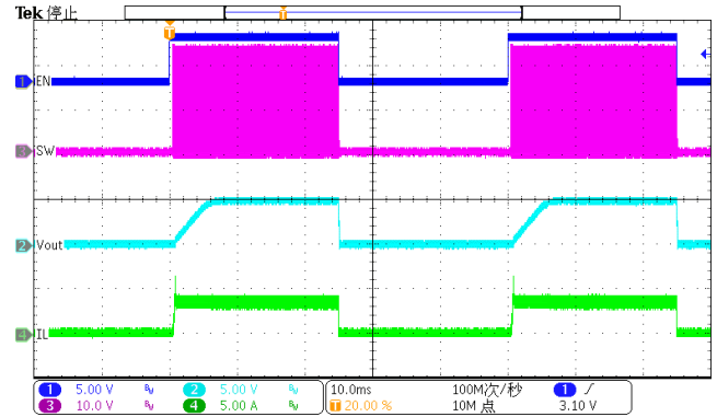
Figure 16. EN toggle ( I_{LOAD}=3.5A )
